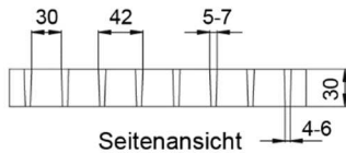
Oldalnézet
